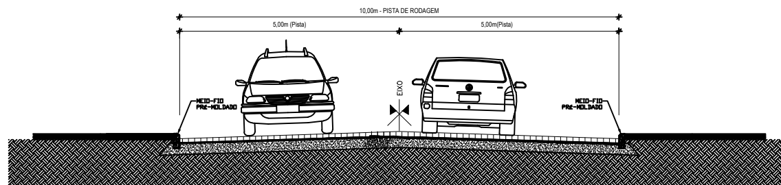
SEÇÃO TIPO DE BLOCO INTERTRAVADO - RUA HELMUTH SCHUETZ
